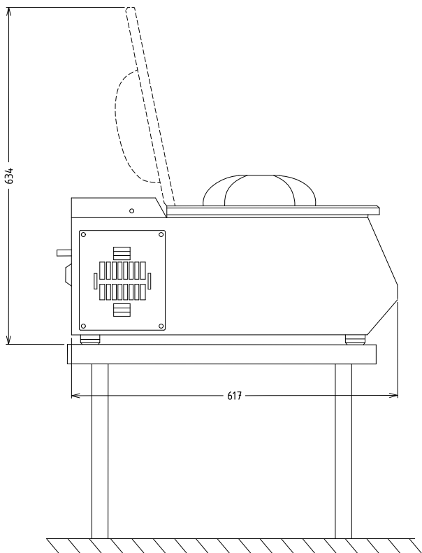
Zij aanzicht
