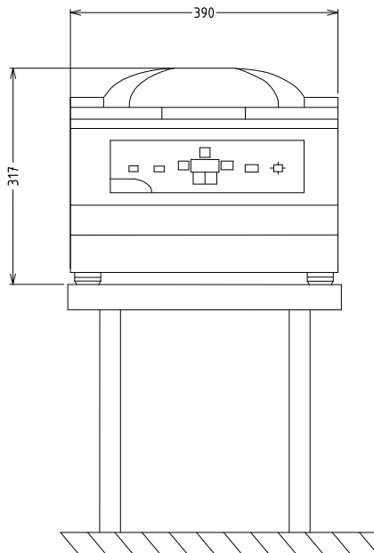
Front aanzicht
